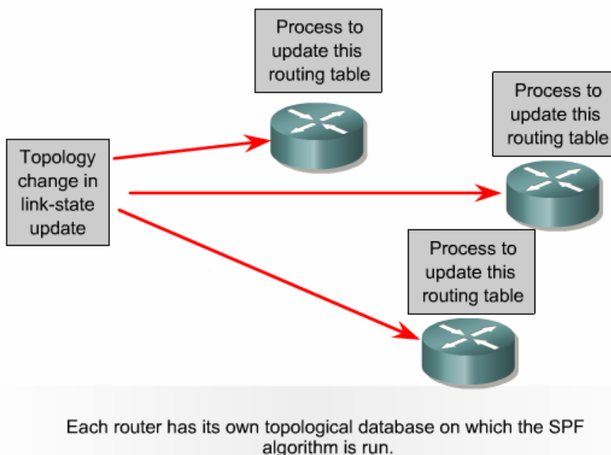
Gambar 6.24 perubahan topologi link-state
