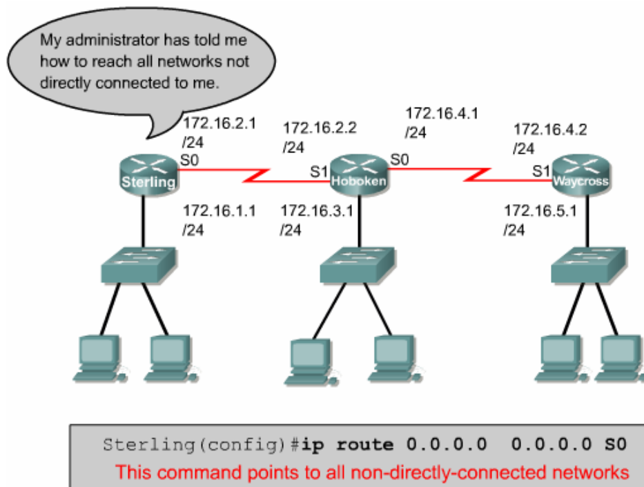
Gambar 6.9 Jaringan yang tidak terhubung langsung
