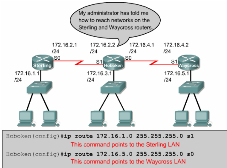
Gambar 6.6 penggunaan interface local sebagai gateway
