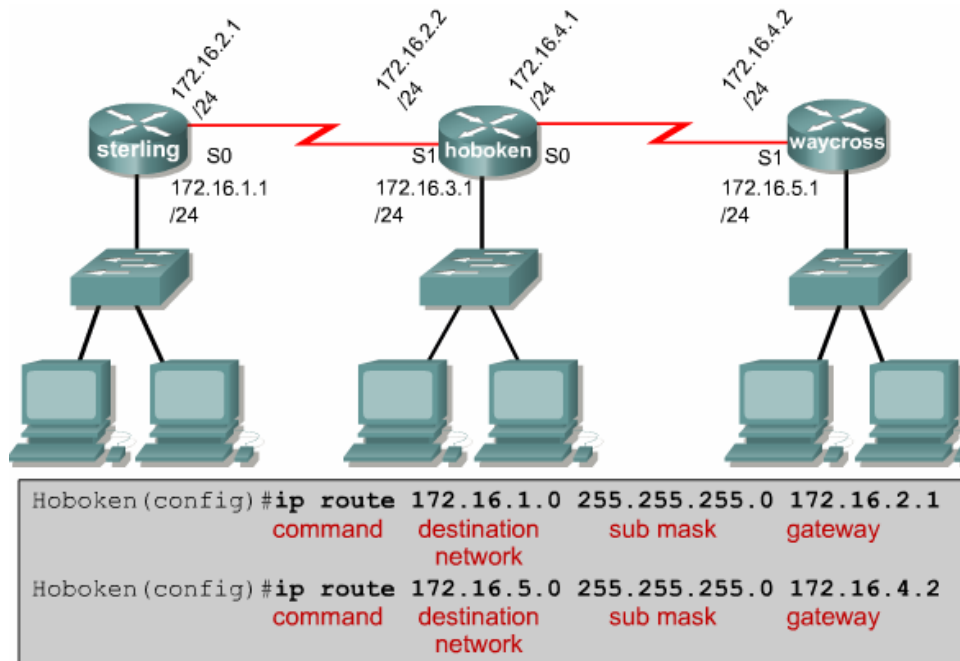
Gambar 6.4 Menentukan Next-hop IP Address
