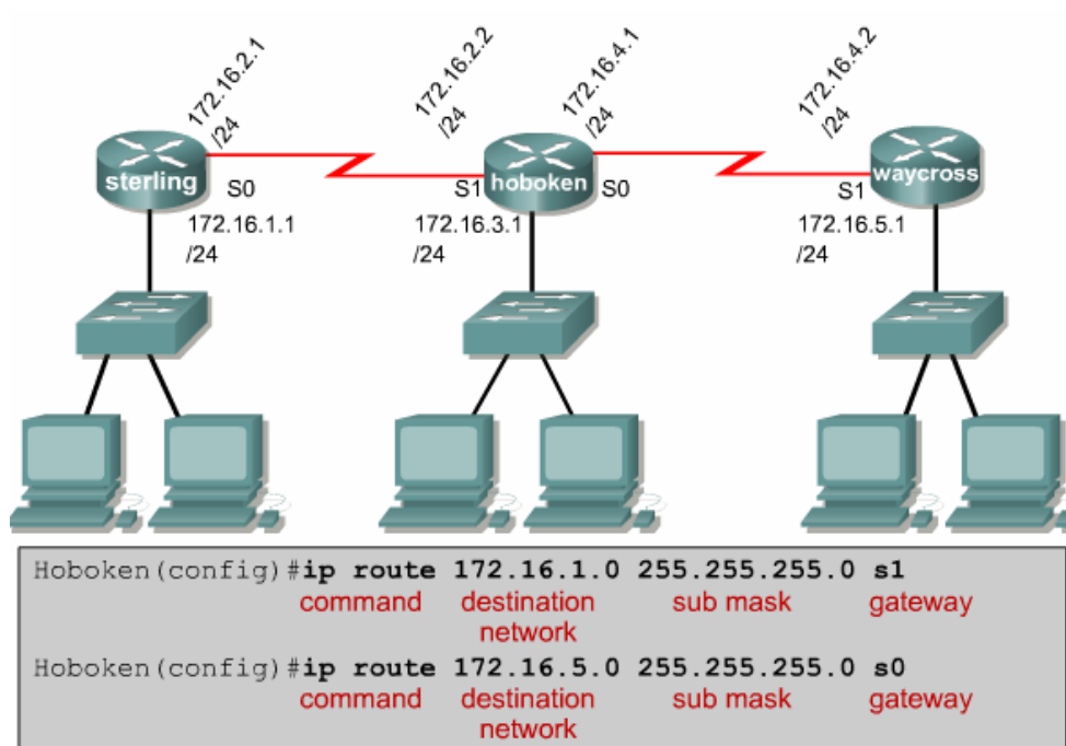
Gambar 6.3 Menentukan outgoing interface
