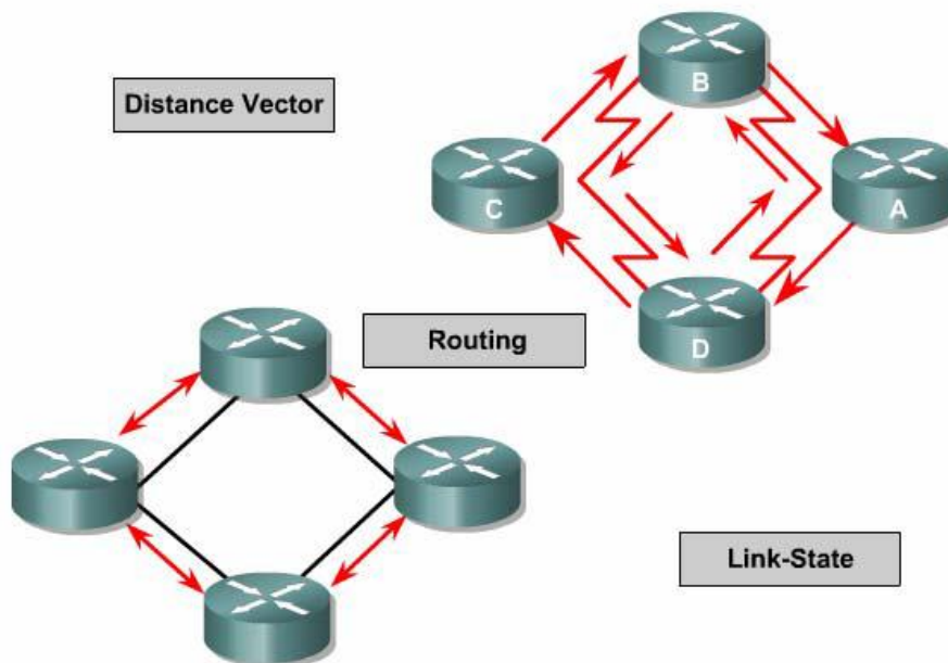
Gambar 6.17 Klasifikasi routing protokol
