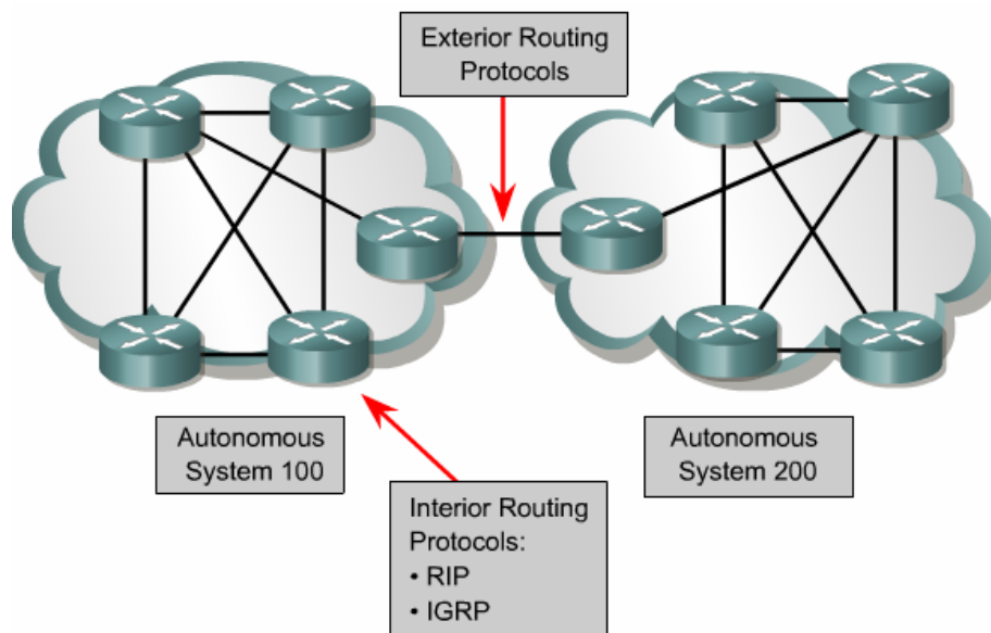
Gambar 6.31 protokol routing interior/eksterior
