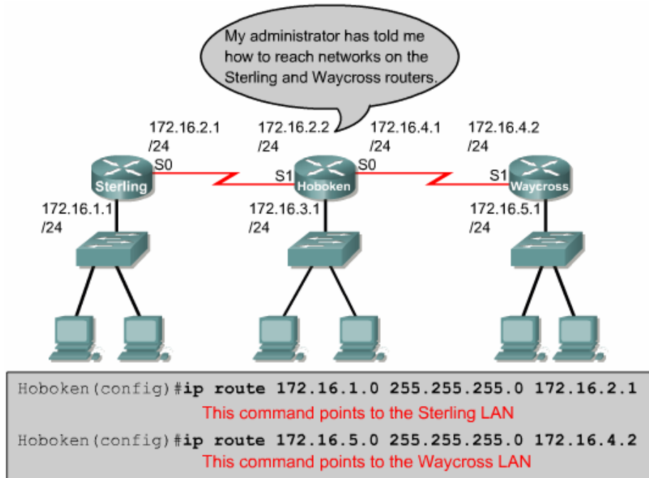
Gambar 6.7 Penggunaan Next-hop
