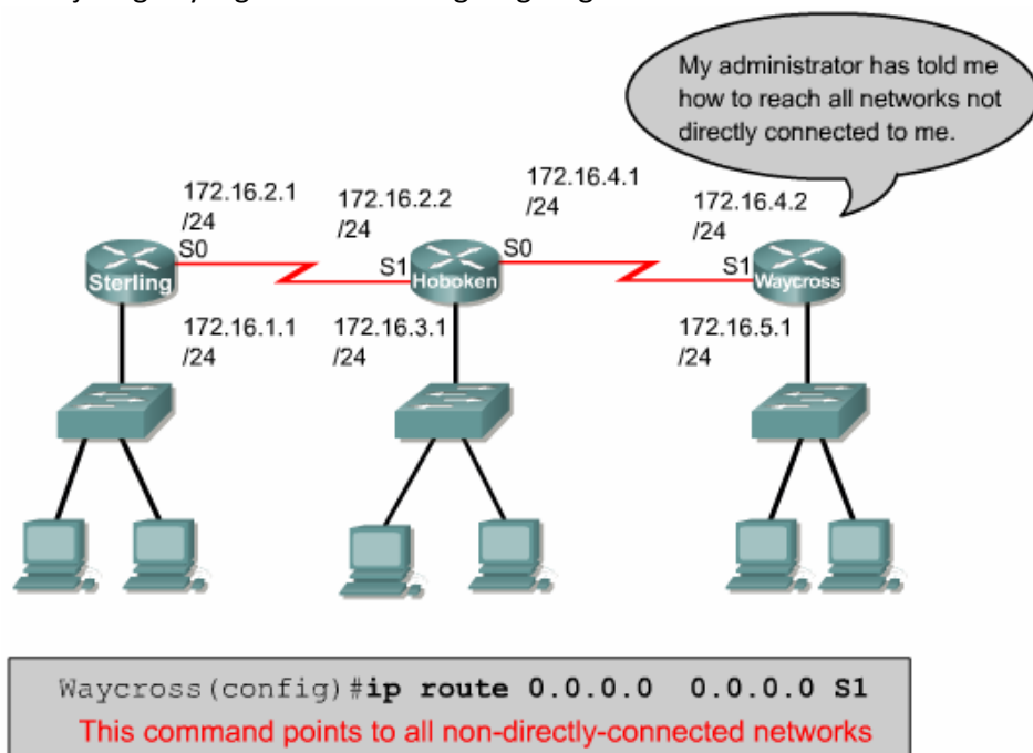
Gambar 6.8 Jaringan yang tidak terhubung langsung
