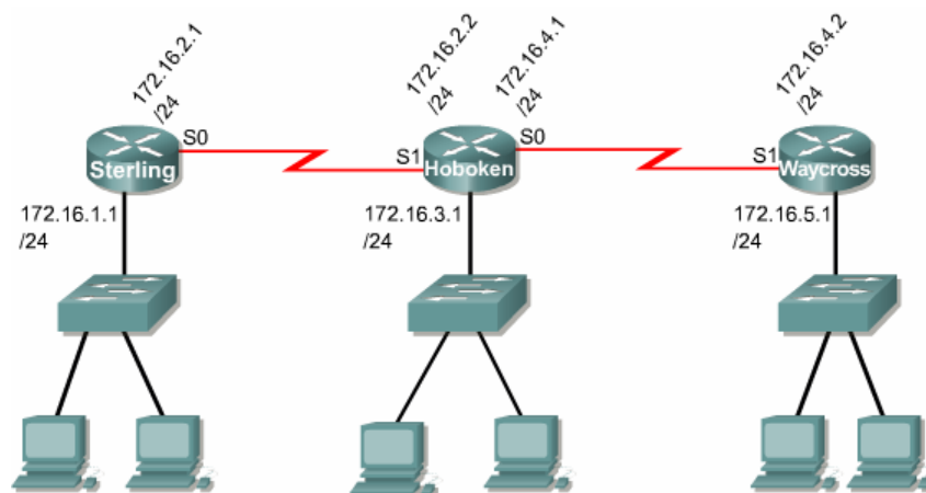
Gambar 6.5 Konfigurasi sederhana dengan 3 Router
